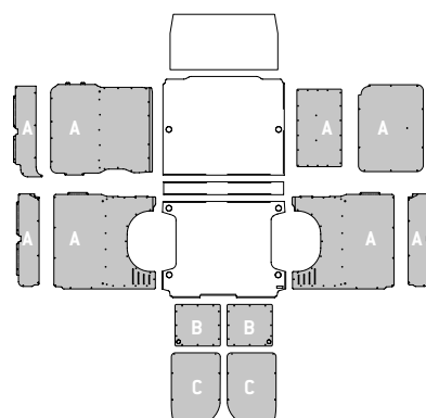
Modello - Modèle L2 H2
