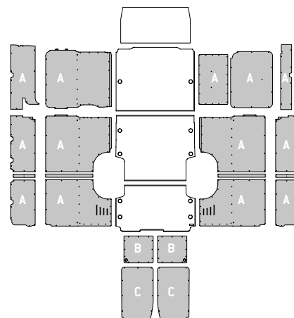
Modello - Modèle L4 H3
