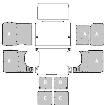
Modello - Modèle L1 H1
