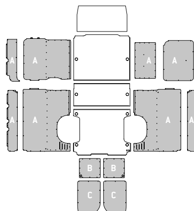
Modello - Modèle L3 H2
