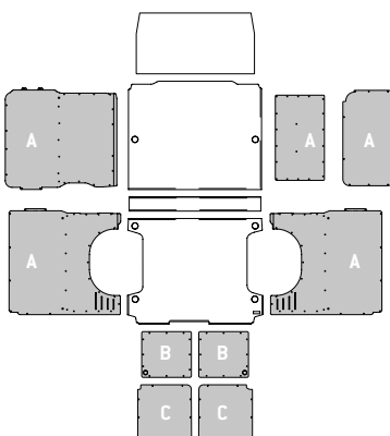
Modello - Modèle L2 H1
